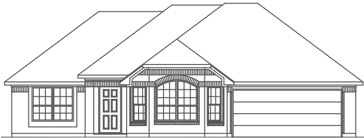
Elev C
