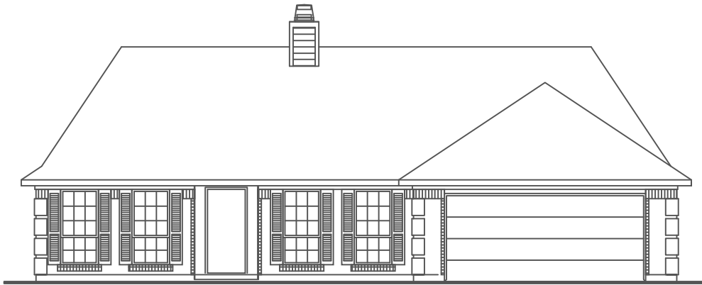
Elev C
