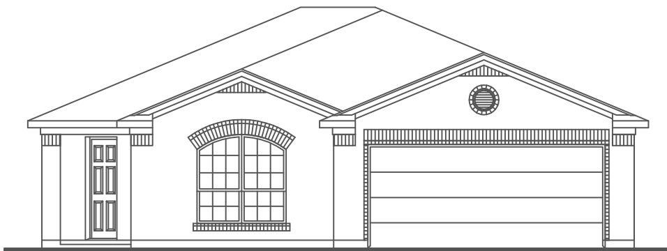
ELEV "B"
